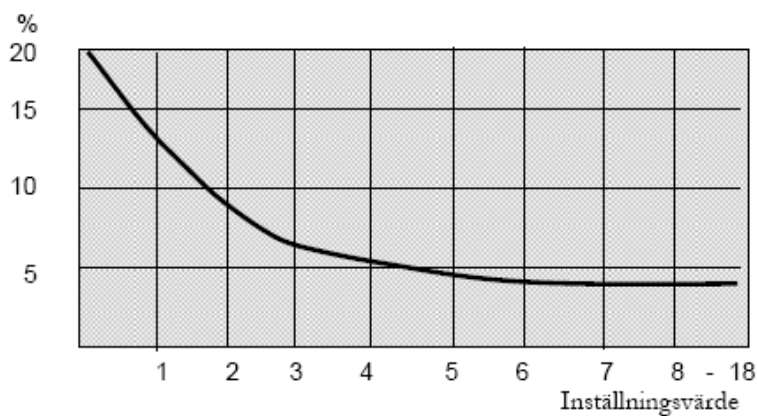
Måtnoggrannhet av Kv värden i %. Ventil 751B DN50 –DN 200
