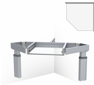
Hörnbänklyft Baselift Corner 6311LA, 45°- 90°, Golvmöglad
